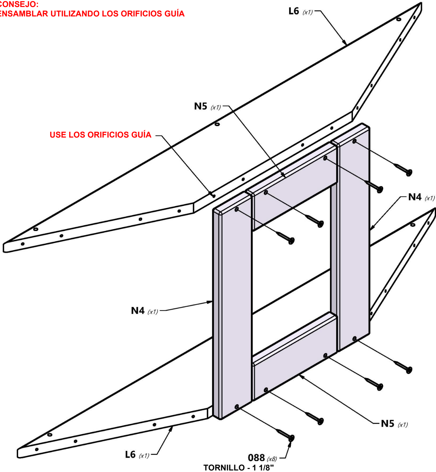
N4 TABLA DE LA VENTANA MIRADOR - W4L14605 (x2) 5/8"x2 3/8"x13 1/8" (16x60x332)
