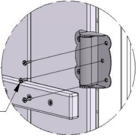
624 (x6) TORNILLO - 5/8"
