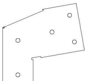
A100326 | SOPORTE DE EXTENSIÓN (x1) DE VIGA DEL COLUMPIO- DERECHA
