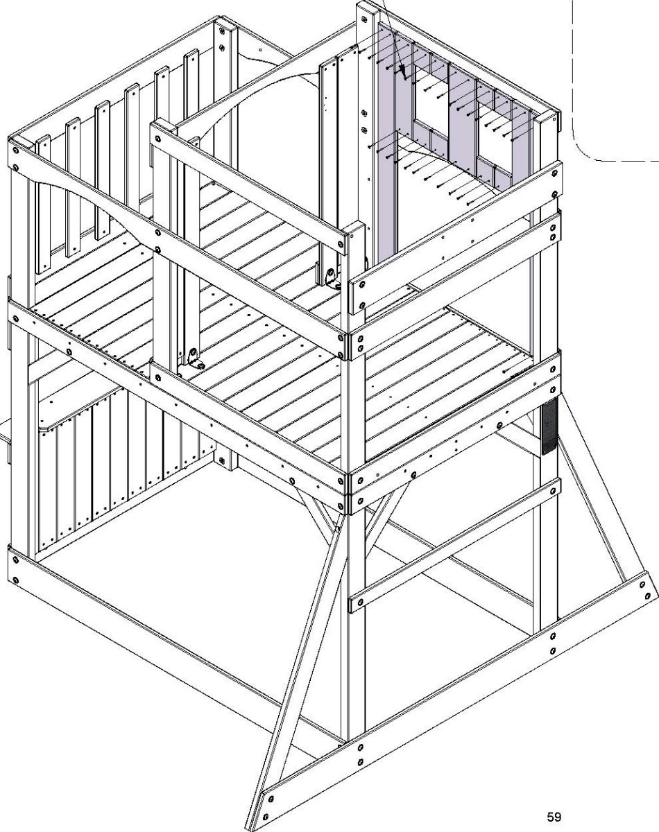
088 (x36) TORNILLO - 1 1/8"
