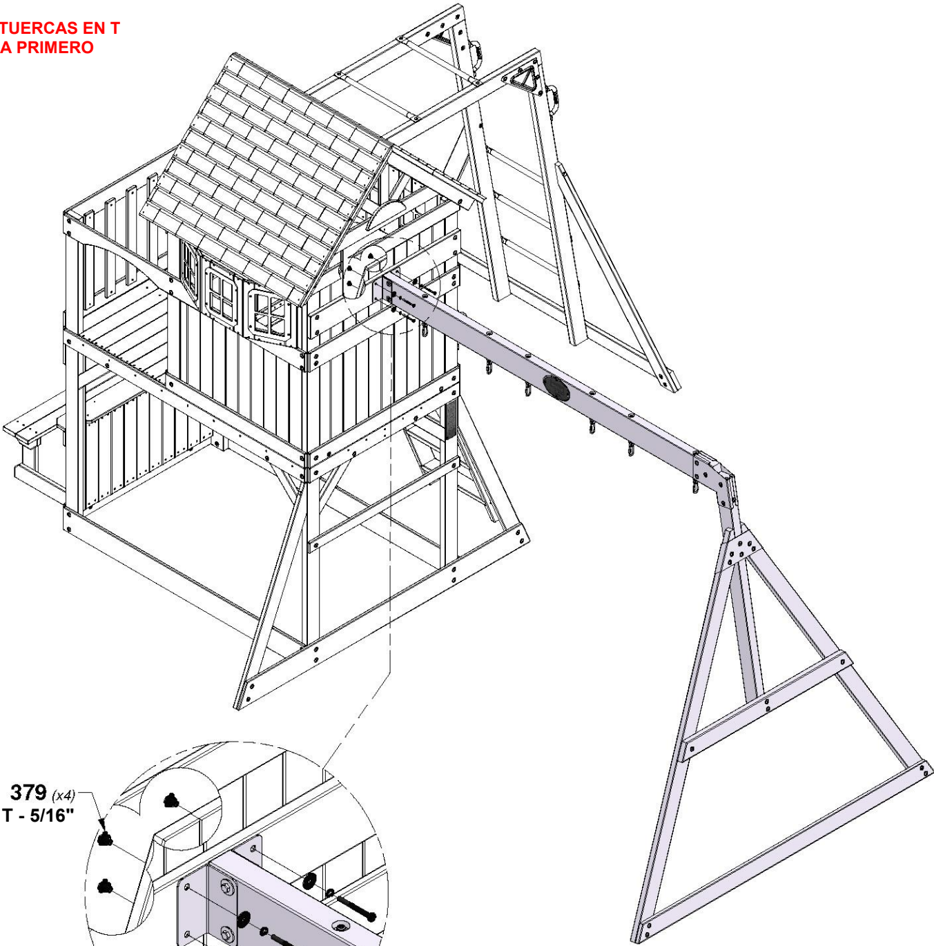
MONTAJE DE LA VIGA DEL COLUMPIO
