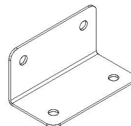
A100140 (x2) | SOPORTE EN ESCUADRA 66x66x127
